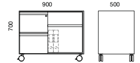
Combo Unit -FF/Open
