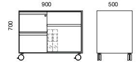
Combo Unit -FF/Open
